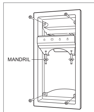
Extracción del bisel del dispensador
