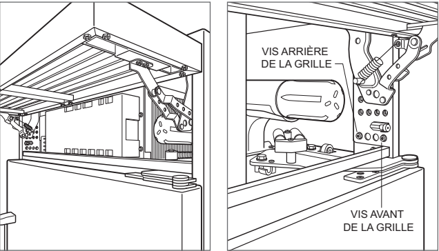
Retrait de la grille
