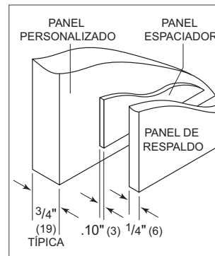
Montaje del panel (vista posterior)
