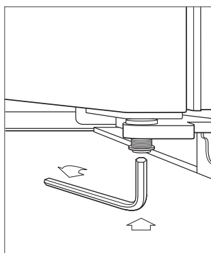
Ajuste de la puerta hacia arriba y hacia abajo
